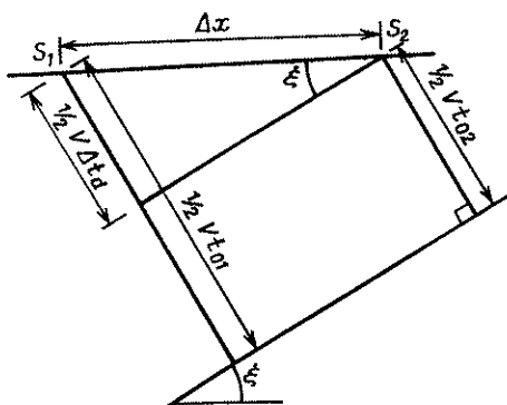
Рис. 3.3. Измерение углового кинематического сдвига между пунктами взрыва или по сейсмическому временному разрезу.
