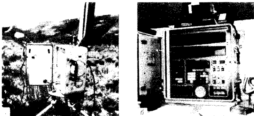
Рис. 5.40. Система Опсейс. Система дает возможность последовательно регистрировать до 4 профилей при 2 расстановках на профиль и 1016 каналов на расстановку. а — выносной телеметрический блок обслуживает 4 группы сейсмоприемников. Сейсмические трассы накапливаются в автономной памяти блока, пока из центрального блока не приходит инструкция об их пересылке. Это дает возможность использовать один радиоканал для многих удаленных блоков, а также обойти ограничения скорости регистрации данных, связанные с протяжкой лент. Система производит автоматическую идентификацию. Взрывник может послать сигнал о взрыве в любой удаленный блок. Если блок перемещается, передается сигнал тревоги, б — программный блок на центральной регистрирующей станции. Клавиатура позволяет оператору вводить данные и инструкции, а панели светящихся диодов выводят информацию для оператора. Связь между центральными и удаленными блоками осуществляется с помощью горизонтально поляризованных волн радиочастотного диапазона. [С разрешения Л. Денэма]
