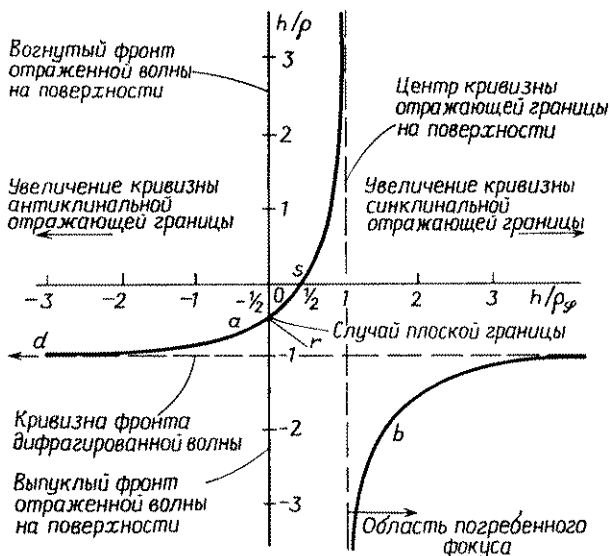
Рис. 4.17. Нормированная кривизна волнового фронта h/\rho на поверхности как функция кривизны отражающей границы h/\rho_{\mathcal{C}} для точечного источника. Буквы d , a , r , s соответствуют кривым рис. 4.18, a , буква b — рис. 4.18, b .
