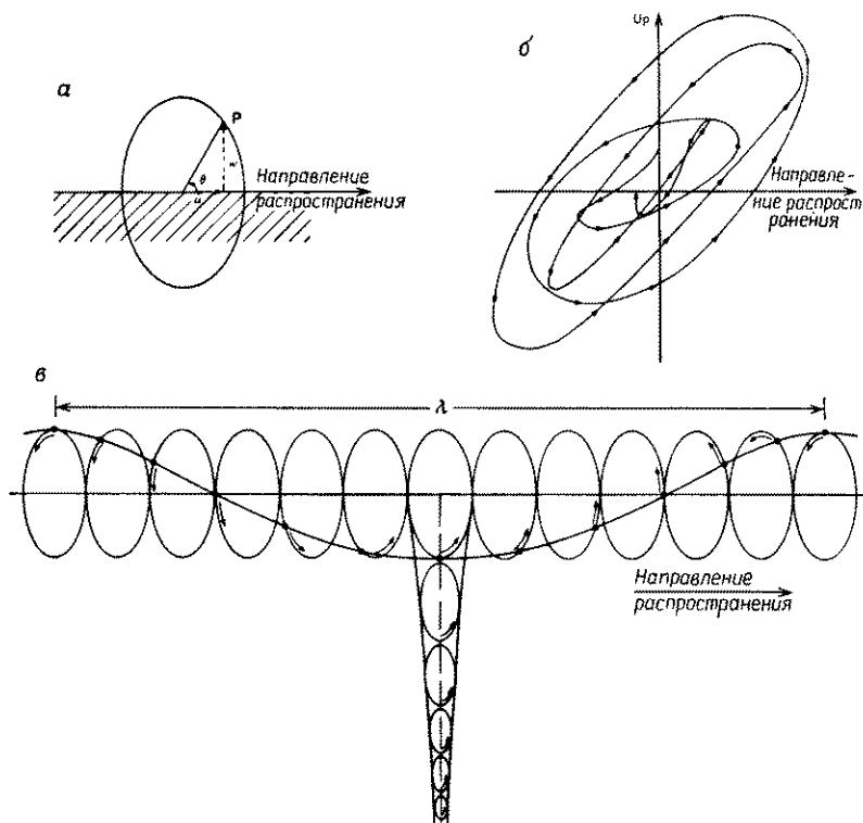
Рис. 2.13 Рэлеевские волны. а — предсказанное движение частицы на поверхности твердого полупространства; б — реальное движение частицы на поверхности Земли [78]; в — поперечный разрез, демонстрирующий движение частиц на поверхности и на глубине для твердого полупространства.
