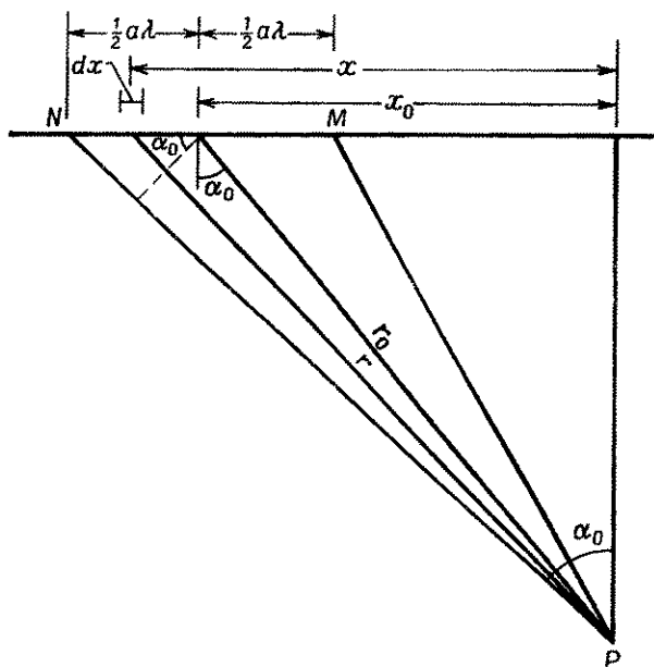
Рис. 5.10. Характеристики непрерывной линейной группы.
