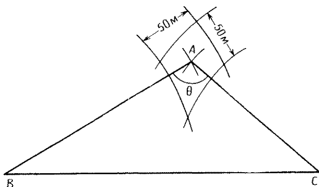
Рис. 5.50. Влияние угла, под которым виден объект с двух береговых станций, на ошибки в определении его местоположения с помощью системы Шоран. \theta — угол видимости, A — подвижная станция, B и C — береговые станции. Точка A может находиться внутри «параллелограмма», образованного четырьмя дугами. (Заметим, что ошибки в определении расстояния даны не в масштабе.)
