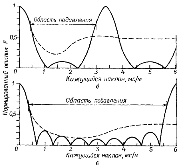
Рис. 5.8. Характеристики направленности группы для колебания с частотой 30 Гц. Эффективная длина группы, от которой зависит ширина главного лепестка, и набор масштабов, показанный на рис. а , одни и те же для всех групп. Положение вторичного (зеркального) лепестка определяется шагом между приборами в группе. Взвешивание увеличивает ослабление сигнала в области подавления. Пунктирные кривые показывают выходной спектр для сигнала с частотным спектром колоколообразной формы, имеющим максимум на частоте 30 Гц и ширину 30 Гц. а — пять сейсмоприемников разнесены по профилю с шагом 10 м; б — пять сейсмоприемников разнесены по профилю с шагом 10 м и весовые множители заданы как 1, 2, 3, 2, 1; в — девять сейсмоприемников разнесены с шагом 5,5 м. [С разрешения фирмы «Шеврон»]
