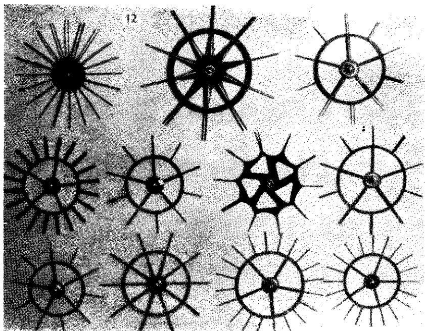
Рис. 1.14. Первые варианты вращающихся устройств для нанесения марок времени (лопастные колеса). Колеса вращались с помощью часового двигателя, в результате чего они пересекали световой луч, создавая тени, служащие марками времени. У наблюдателей часто имелись колеса своих собственных конструкций, что отличало записи друг от друга. (Сфотографировано в Музее геофизического общества Хьюстона.)
