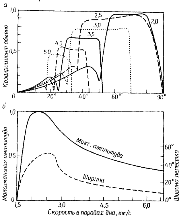
Рис. 5.66 Обменные эффекты на границе жидкость — твердое тело. а — коэффициент обмена в функции угла падения в воде; параметр кривых — скорость в породах под поверхностью дна (в км/с); б — максимальная амплитуда и ширина главного лепестка в зависимости от скорости в донных породах [200].
