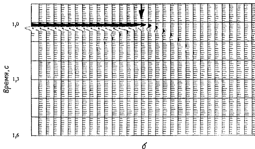
Рис. 2.23. Сейсмический эффект от полуплоскости [206]. а — модель; б — рассчитанный сейсмический разрез при совмещенных источниках и сейсмоприемниках. Острые стрелки указывает расположение края полуплоскости.
