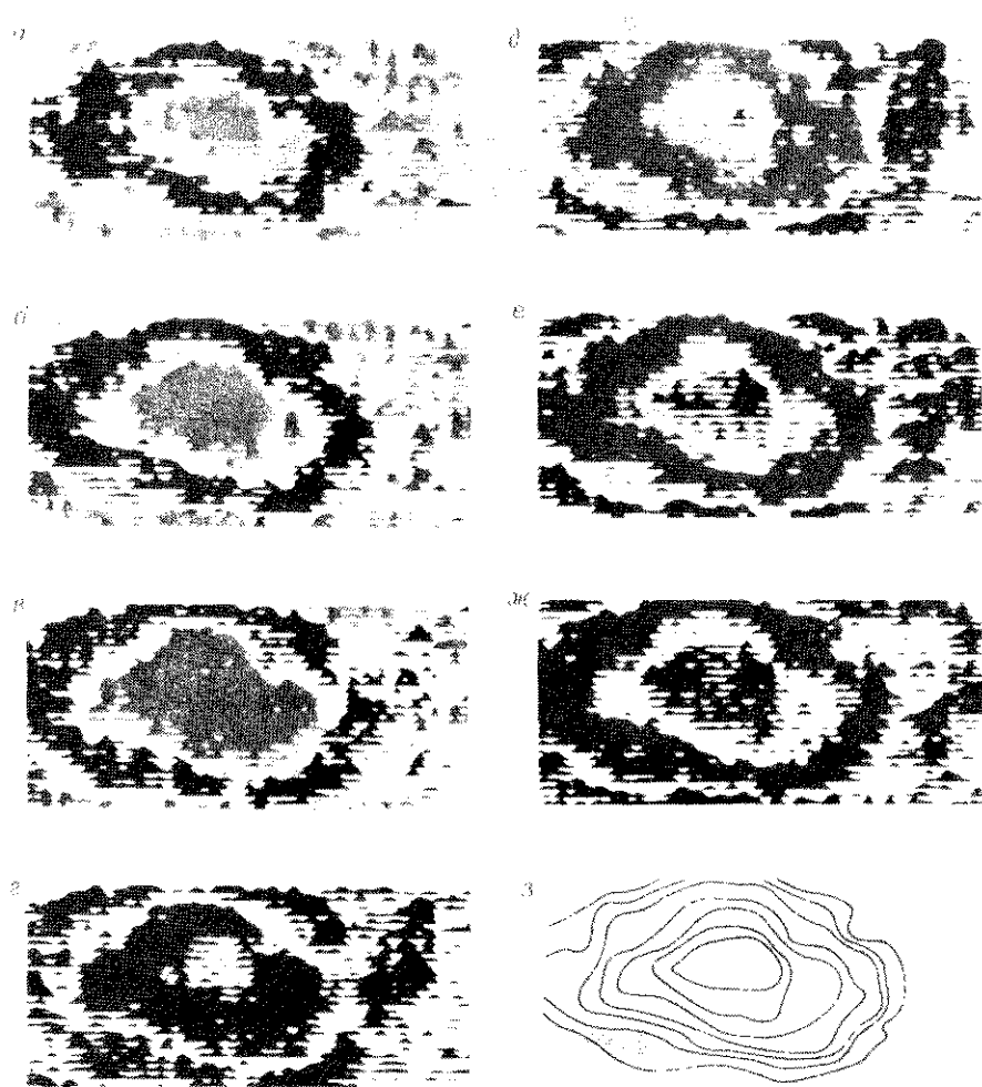
Рис. 5.36. Набор карт временных сечений. Площадь сечений 3,6 \times 8,0 км. От а до ж даны карты при t = 1,580 \div 1,604 с с интервалом 4 мс; з — карта изохрон, построенная путем прослеживания изолиний каждого сечения от а до ж , начиная от внешней изолинии центральной области на самом верхнем срезе ( а ). [С разрешения GSI]
