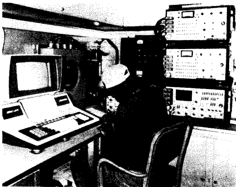
Рис. 5.37. Цифровая полевая аппаратура, смонтированная в автомобиле; регистрирующая система включает некоторые специальные устройства для обработки данных. [С разрешения TI]
