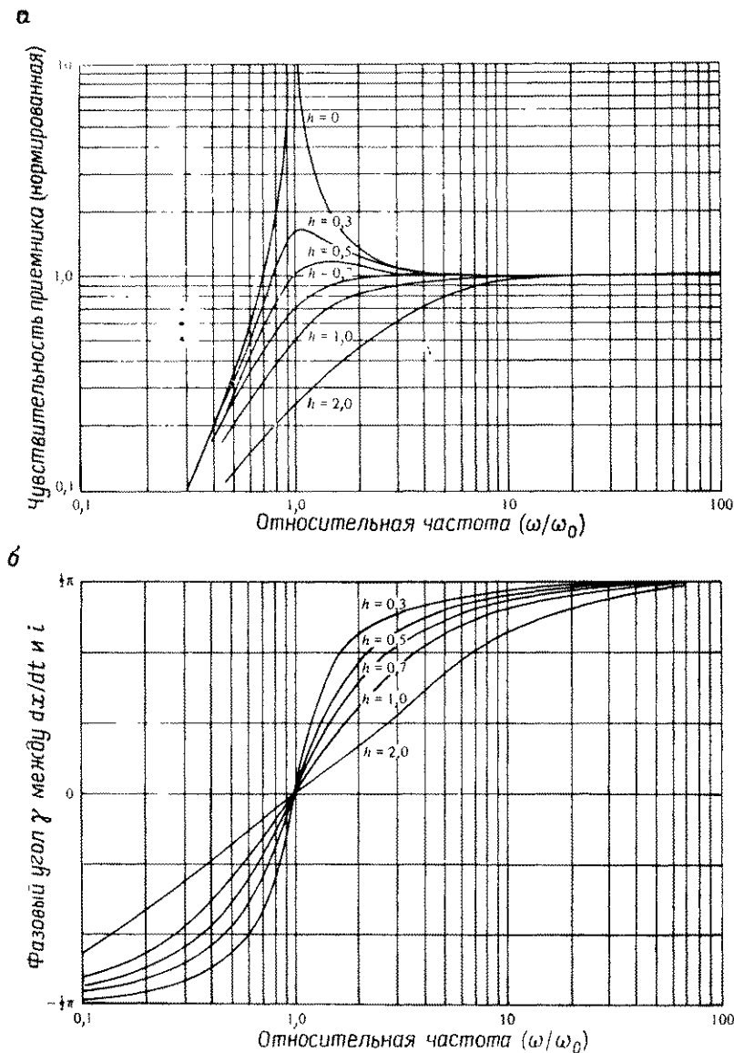
Рис. 5.31. Характеристики сейсμοприемника в зависимости от коэффициента затухания h [45]. а — амплитудно-частотная характеристика; б — фазовая характеристика.
