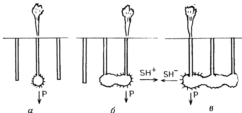
Рис. 5.65. Метод Сисслера: а — взрыв в центральной скважине генерирует в основном P -волны; б — благодаря асимметрии среды, созданной взрывом в центральной скважине, при взрыве в правой скважине наряду с P -волнами излучаются также SH -волны; в — при взрыве в левой скважине образуются P -волны и SH -волны противоположной по отношению к предыдущему случаю полярности. [С разрешения CGG]
