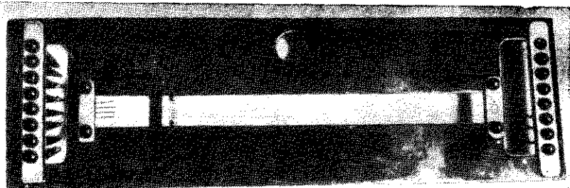
Рис. 1.8. «Гриф» струнных гальванометров. Токи, проходящие через тонкие проволоочки (некоторые из них на длинном «грифе» разорваны), натяжение которых обеспечивается маленькими пружинками, заставляют проволоочки отклоняться в магнитном поле. Тени от проволоочек фиксируются на фотобумагу. Запись, сделанная с помощью струнных гальванометров, приведена на рис. 1.15, д. (Сфотографировано в Музее геофизического общества в Хьюстоне.)
