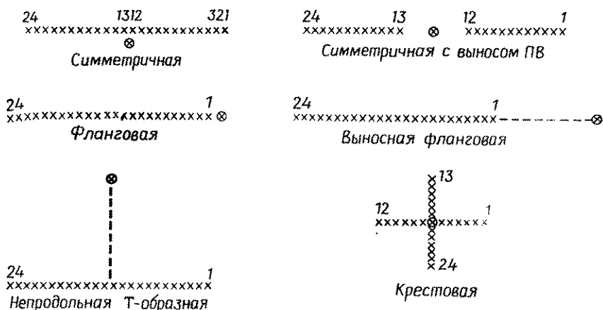
Рис. 5.6. Типы расстановок в методе отраженных волн. Крестики и крестики в кружках означают положение групп источников и пунктов взрыва соответственно.
