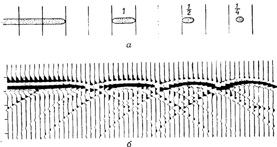
Рис. 4.25. Отражение от тонкого пласта ограниченной протяженности (протяженность выражена в долях ширины зоны Френеля) [129]. a — разрез модели, расстояние между вертикальными прямыми равно диаметру зоны Френеля; б — сейсмический разрез.
