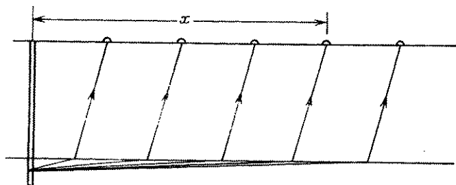
Рис. 5.59. Изучение ЗМС с помощью преломленных волн.
