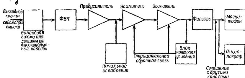
Рис. 5.32. Аналоговая сейсмическая станция: а — переносная станция [с разрешения фирмы TI]; б — блок-схема аналогового сейсмического усилителя.
