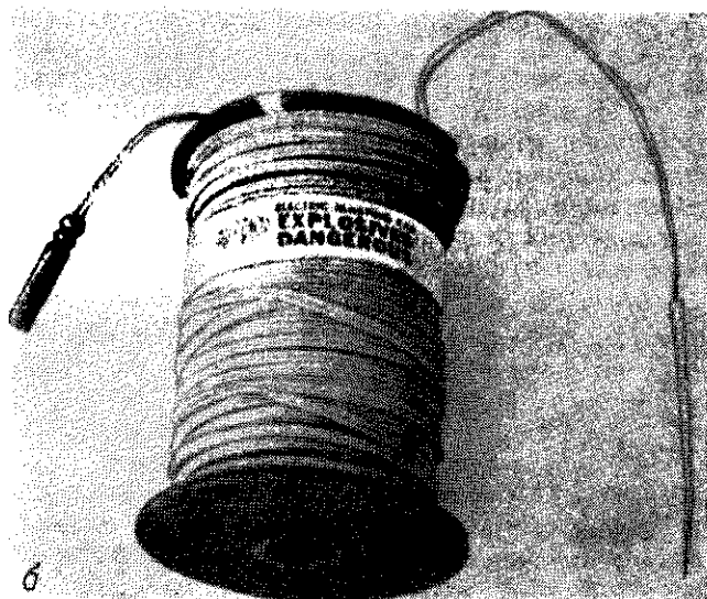
Рис. 5.24. Взрывчатые вещества для сейсмических исследований а — цилиндрические шашки Нитрамон, соединенные концами; б — электродетонатор. [С разрешения фирмы «Дю Пон»]
