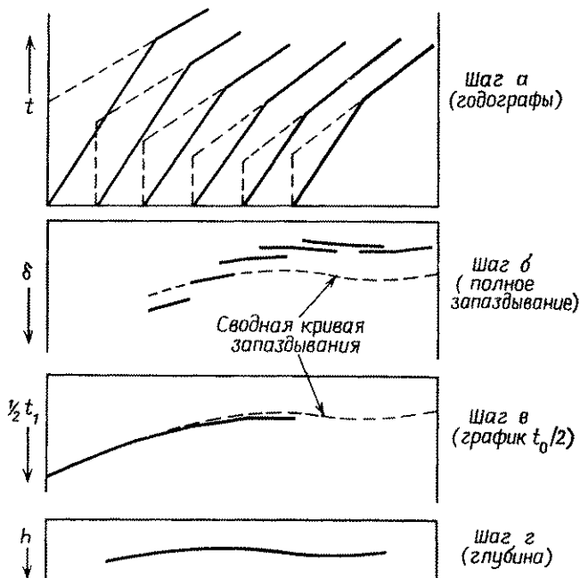
Рис. 6.13. Интерпретация профилей, отработанных в одном направлении, по методу Виробека [225].
