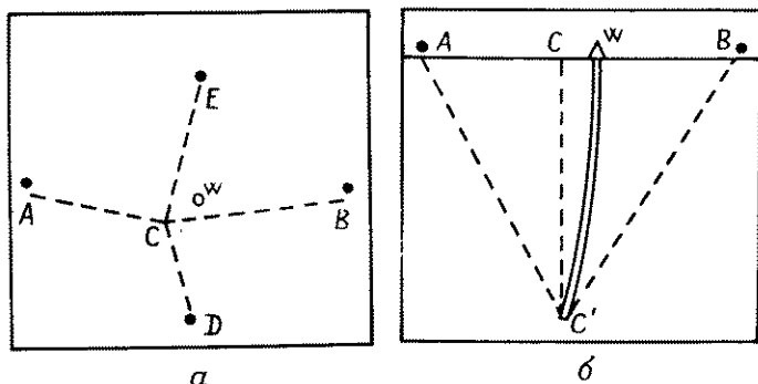
Рис. 3.26. Картирование искривленной скважины по измерению времени пробега до сейсмоприемника, расположенного в точке C внутри скважины [15]. a — вид сверху; b — вертикальный разрез по AWB .
