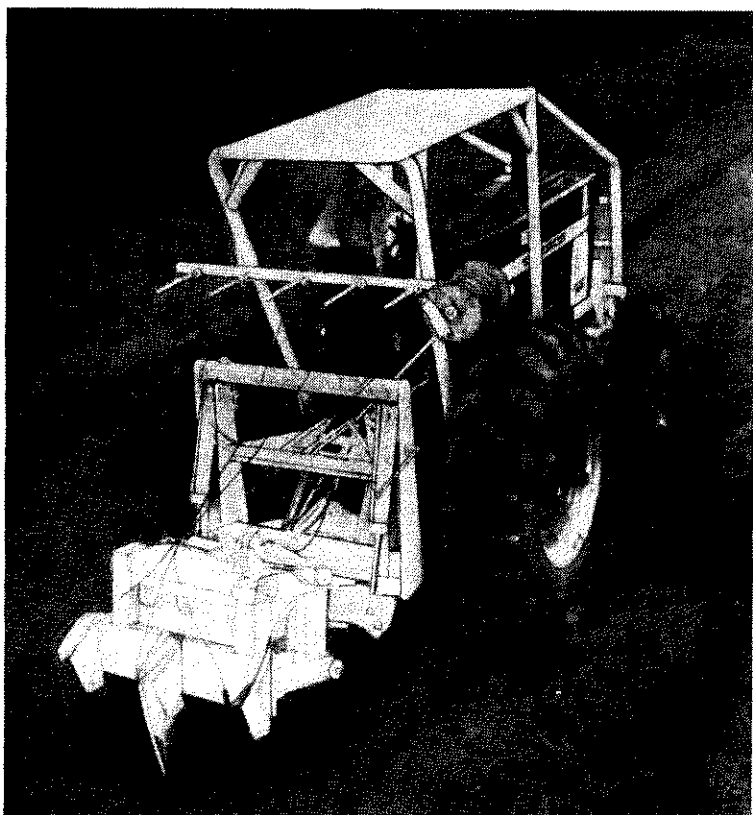
Рис. 5.25. Плуг для укладки детонирующего шнура. Шнур опускается вниз по трубам, расположенным позади лопастей, которые вибрируют при продвижении вперед, укладывая шнур на глубину от \frac{2}{3} до 1 м под поверхность. [С разрешения «Примакорд сервисес»].
