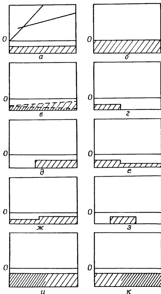
Рис. 3.25. Годографы в случае различных двухслойных моделей. Рисунок составлен по иллюстрациям к статье [15], первой публикации на английском языке по сейсмическому методу. В верхней части (выше точки O ) каждой схемы оставлено место для построения годографов соответственно моделям, представленным на разрезе ниже точки O . Схема a иллюстрирует, что именно требуется сделать. В схеме б предлагаются две альтернативы, поэтому должны быть изображены два набора кривых. В схемах и и к предполагается, что скорости меняются в горизонтальном направлении пропорционально плотности штриховки; в каждом из этих случаев скорость в пределах заштрихованного участка больше, чем в вышележащем слое.
