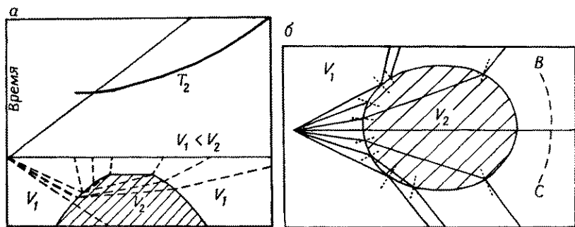
Рис. 2.33. Пути пробега волн через соляной купол согласно закону Снеллиуса [15]. а — вертикальный разрез; б — вид в плане.
