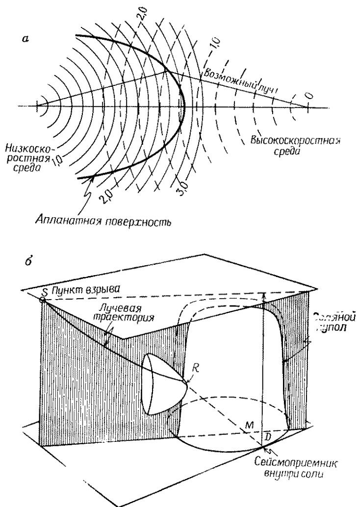
Рис. 6.6. Оконтурирование соляного купола с использованием сейсмоприемника внутри соли [62]. a — вид апланатной поверхности в плане; b — изометрическое изображение лучевой траектории и параболоида апланатной поверхности.
