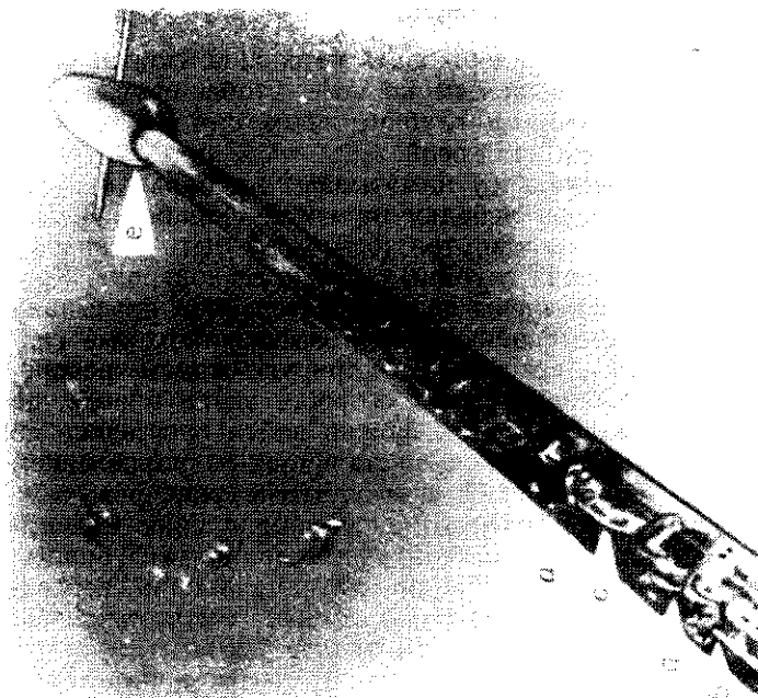
Рис. 5.49. Схема и фотография сейсмической косы. Пластмассовые разделители a соединены тремя эластичными проводниками b ; связка электрических проводов c проходит сквозь отверстия разделителей. Гидрофон помечен буквой d . Сейсмическая коса помещается в мягкую пластмассовую оболочку, наполненную жидкостью, которая обеспечивает косе нейтральную плавучесть. Устройства для регулирования глубины погружения ( e ) закреплены на косе. [С разрешения «Сейсмик энджиниринг»]
