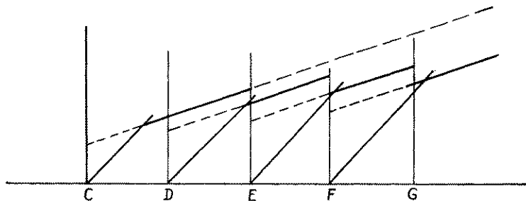
Рис. 6.3. Система индивидуальных годографов МПВ в случае одной преломляющей границы
