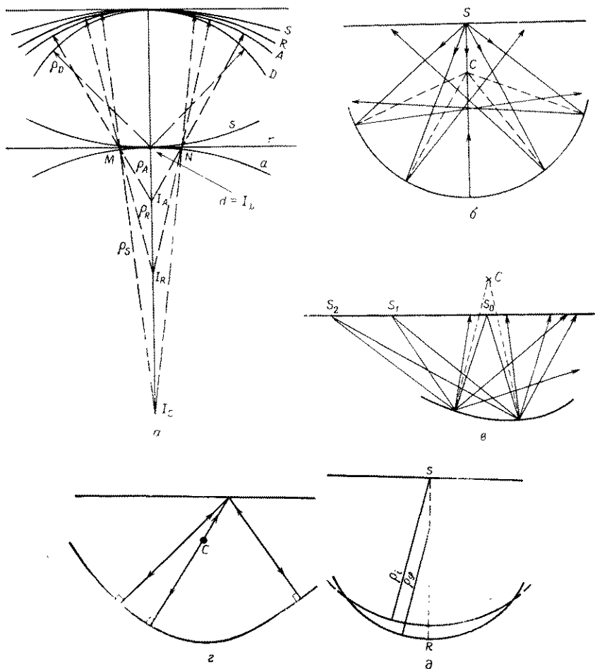
Рис. 4.18. Эффект кривизны отражающей границы. a — влияние на кривизну волнового фронта перехода отражающей границы от антиклинального типа к синклинальному: d — точка дифракции, a — антиклиналь, r — плоская отражающая граница, s — синклиналь. Им соответствуют волновые фронты D , A , R , S , мнимые источники I D , I A , I R , I S и радиусы кривизны \rho_D , \rho_A , \rho_R , \rho_S . b — траектории лучей, проходящих через область фокусировки, когда центр кривизны C лежит ниже поверхности e — для удаленных трасс траектории отраженных волн S 1 и S 2 проходят через фокус даже тогда, когда для ближних трасс эти траектории S 0 не проходят через фокус z — отражения от ряда точек отражающей границы, когда ее кривизна меняется, d — волновой фронт с радиусом \rho_i падает на отражающую границу с радиусом кривизны \rho_s , когда \rho_i > \rho_s .
