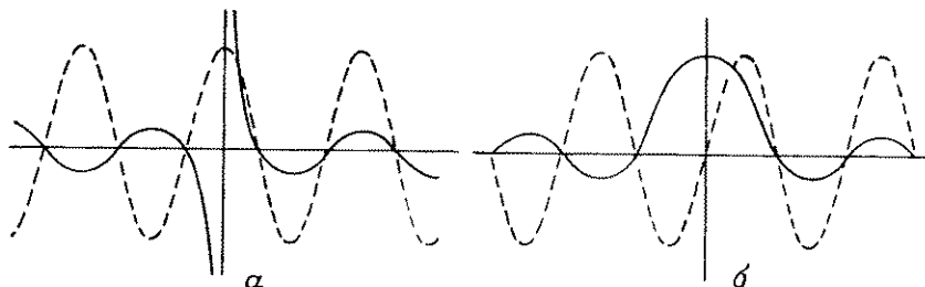
Рис. 4.21. Сравнение поведения сферической (сплошные кривые) и плоской (пунктирные кривые) волн, проходящих через фокальную точку. a — член \cos(\omega r/V) в выражении (4.8); b — член \sin(\omega r/V)/(\omega r/V) .
