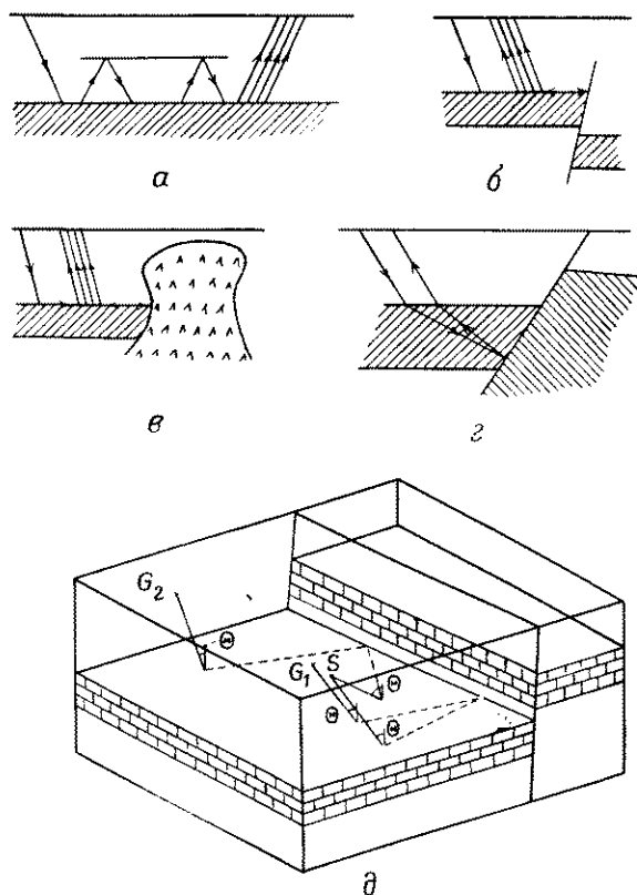
Рис. 4.16. Отраженно-преломленные волны, а — многократно-отраженные преломленные волны; б , в , г — преломленные волны, отраженные от сбросов и соляных куполов; д — изометрическая схема преломленных волн, отраженных от уступа преломляющей поверхности в стороне от профиля; показаны траектории от источника S до приемников G 1 и G 2 , пунктирные линии соответствуют траектории головной волны по кровле преломляющего слоя.
