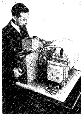
Рис. 1.18. Сонограф Рибера, 1936 г. Получаемые в поле данные регистрировались на пленке способом переменной плотности. При воспроизведении суммировался весь свет, проходящий через щель, и создавалась единая выходная трасса. Изменяя угол установки щели, можно усиливать волны с различными углами выхода (дающие так называемый кажущийся угол наклона; см. § 3.1.2), причем каждый угол установки щели приводит к получению одной дополнительной трассы. Таким образом, на получаемой в итоге записи амплитуда сигнала изображается в виде зависимости угла выхода от времени вступления. (Два снимка из рекламных объявлений в «Geophysics», т. 1 и 2.)
