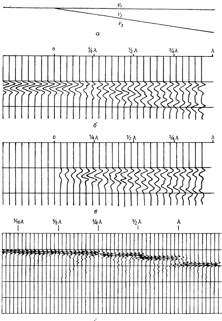
Рис. 4.22. Синтетические сейсмограммы отраженных волн, иллюстрирующие вертикальную разрешенность [181]. a — модель выклинивающегося слоя; б — отражение от слоя при V_3 > V_2 > V_1 (указана толщина слоя в долях преобладающей длины волны); в — отражение от тонкого клина, заключенного в однородной среде ( V_3 = V_1 \neq V_2 ); г — отражения от границы, нарушенной разломами (указано смещение по разломам в долях преобладающей длины волны).
