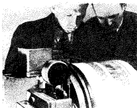
Рис. 1.18. Сонограф Рибера, 1936 г. Получаемые в поле данные регистрировались на пленке способом переменной плотности. При воспроизведении суммировался весь свет, проходящий через щель, и создавалась единая выходная трасса. Изменяя угол установки щели, можно усиливать волны с различными углами выхода (дающие так называемый кажущийся угол наклона; см. § 3.1.2), причем каждый угол установки щели приводит к получению одной дополнительной трассы. Таким образом, на получаемой в итоге записи амплитуда сигнала изображается в виде зависимости угла выхода от времени вступления. (Два снимка из рекламных объявлений в «Geophysics», т. 1 и 2.)
