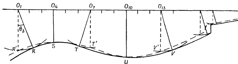
Рис. 5.62. Искажение разреза из-за неучета сейсмического сноса.
