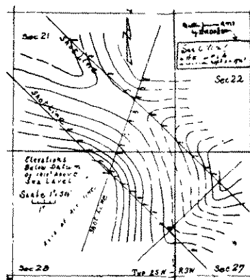
Рис. 1.3. Первое применение сейсмографа для записи отраженных волн в сейсморазведке [171]. а —две сейсмограммы, записанные в сентябре 1921 г.; буквой Е отмечен момент взрыва, Р —отражение от известняков Вайола, ВР —воздушная волна (акустический датчик взрывной волны). б —первый глубинный разрез, полученный по данным наблюдений в Вайнз-Бранч, шт. Оклахома, США, 9 августа 1921 г. в —первая сейсмоструктурная карта (вблизи Понка-Сити, Оклахома, сентябрь 1921 г.).
