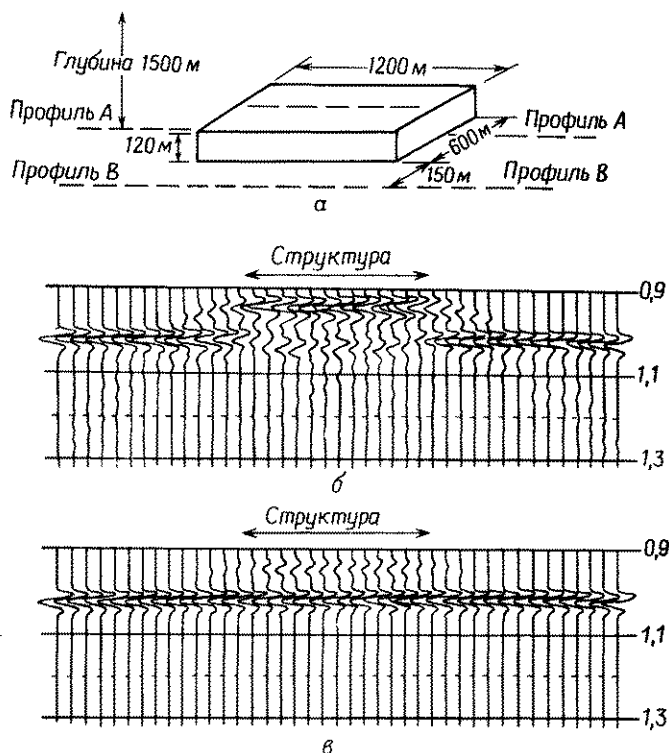
Рис. 4.28. Профиль через коробкообразную структуру. Расстояние между трассами 85 м, радиус зоны Френеля 280 м для частоты 30 Гц. [С разрешения фирмы «Геовест»] а — модель; б — профиль А через кровлю структуры; в — профиль В , не пересекающий структуру.
