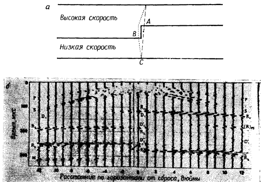
Рис. 4.8. Эффект ступени [7]. а — модель; б — запись в случае центральной расстановки приемников с источником над ступенью: P — прямая волна, S — поверхностная, R_t и R_b — волны, отраженные от верхней и нижней поверхности ступени, R_b — отраженные волны от основания модели, D_1 и D'_1 — дифрагированные волны на верхнем и нижнем краях ступени, M — кратные отражения, (R)_{ps} — обменная волна. Имеется и дифрагированная волна-призрак ( D'_1 ), которая продолжает отражение R_b за центр расстановки.
