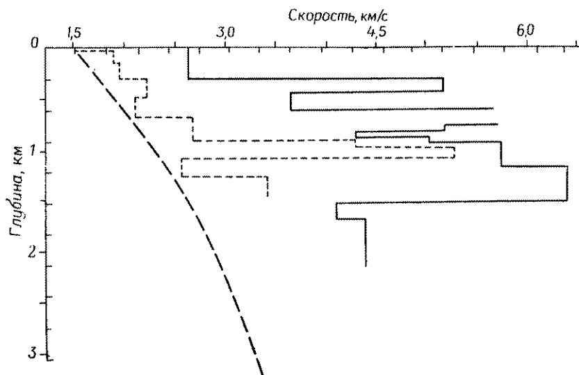
Рис. 6.23. Зависимость скорости от глубины по скважинам в Иллинойсском бассейне (сплошная линия), в Яванском море (пунктир) и на побережье Мексиканского залива в районе шт. Луизиана (штриховая кривая).
