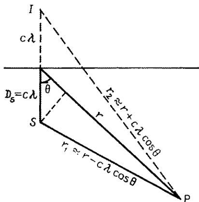
Рис. 4.11. Направленность системы источник плюс волна-спутник. S — источник, I — мнимый источник (порождающий волну-спутник), P — точка наблюдения.
