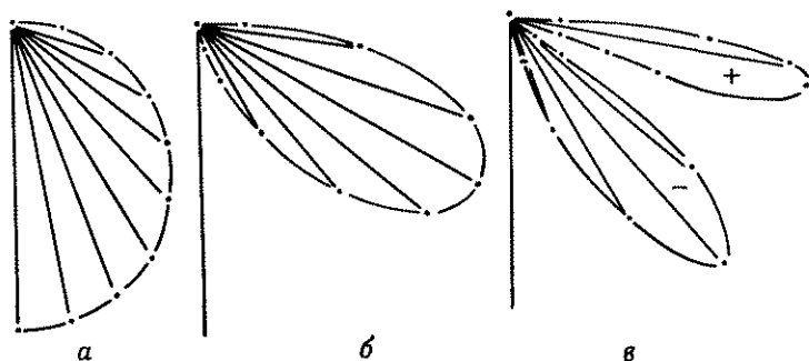
Рис. 4.33. Диаграммы направленности гармонического источника, расположенного на различных глубинах под свободной поверхностью ( h — глубина в долях длины волны): a — h = 0,1 ; b — h = 0,5 ; v — h = 1,0 [214].
