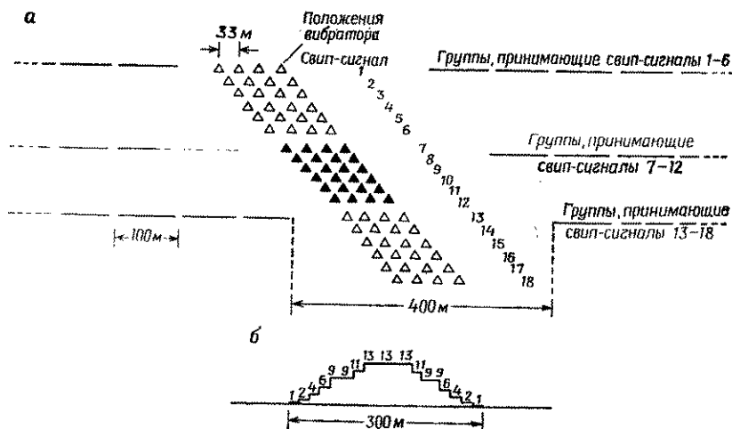
Рис. 5.13. Схема наблюдений при использовании поверхностных источников. Четыре установки Вибросейс (или других источников), разнесенные на 33 м, двигаются одна за другой слева направо вдоль профиля, производя излучения одновременно через каждые 17 м. Во избежание наложения треугольников на рисунке положения вибраторов во время последовательных излучений смещены по вертикали. Шесть последовательных свип-сигналов суммируются (синфазное суммирование — см. § 5.4.9) для получения одной выходной полевой записи. Четыре центральные группы не используются, так как их записи слишком зашумлены работой вибраторов. После излучения 6-го свип-сигнала к регистрирующей станции подключается следующая по ходу группа, образуя активные группы, показанные на центральной горизонтальной линии рис. а; эти группы регистрируют свип-сигналы с 7-го по 12-й, излучаемые вибраторами в положениях, отмеченных зачерченными треугольниками. а — положение источников и активных групп сейсмоприемников для последовательных свип-сигналов; б — эффективная комбинация групп, цифры показывают число составляющих свип-сигналов (результат свертки линейной группы с суммарной характеристикой направленности шести свип-сигналов с 1-го по 18-й; см. § 8. 1.2 и задачу 8.13, а).
