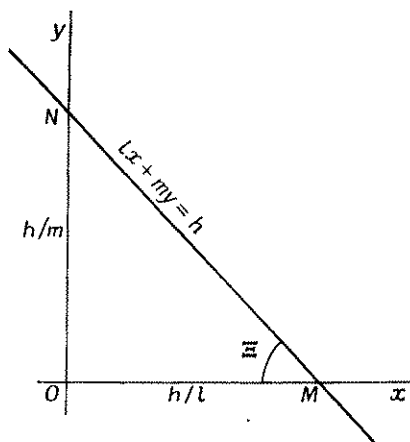
Рис. 3.7. Определение угла простирания.
