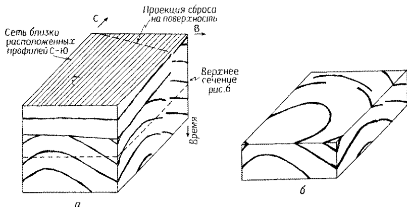
Рис. 5.35. Трехмерные данные, полученные с помощью сети близко расположенных профилей, ориентированных в направлении С—Ю. а — изометрический чертёж объема, занимаемого этими данными; показан разрез на восточном окончании серии профилей, а также разрез по линии В—З, построенный по самым южным трассам каждого профиля; б — изометрический чертёж сети тех же данных со снятой верхней частью разреза; верхняя поверхность представляет собой карту временного сечения (Сейскроп).
