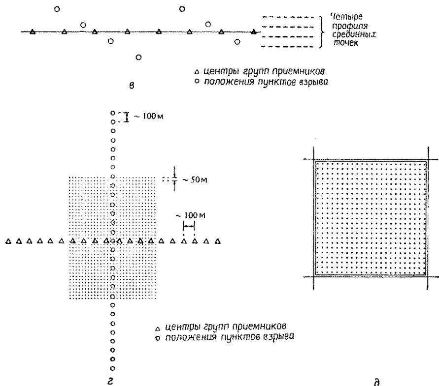
Рис. 5.18. Методика трехмерных наблюдений. а — положение корабля и 48 приемных групп, нанесенное в каждом 25-м пункте взрыва; б — использование параванов для отведения источников в стороны от курса корабля с целью получения двух профилей срединных точек; в — расстановка по методике широкого профиля; г — блоковая расстановка; д — расстановка по методике «Сейслуп» с расположением сейсмоприемников и пунктов взрыва по периметру площади (срединные точки показаны маленькими точками; 40 групп сейсмоприемников и 40 пунктов взрыва можно расположить с интервалом 160 м по четырем сторонам квадрата с длиной стороны 1,6 км).
