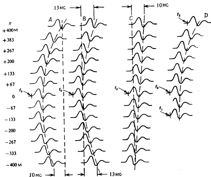
Рис. 3.4. Связь между нормальным и угловым кинематическим сдвигом. Для сейсмограмм A , B и C t_0 = 1,000 с, V = 2500 м/с. Для сейсмограммы D t_0 = 1,225 с, t_1 = 1,223 с, t_2 = 1,242 с, V = 2800 м/с.
