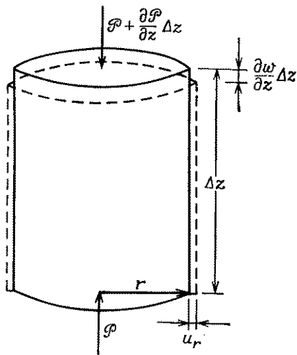
Рис. 2.15. Изменения в среде при прохождении трубной волны.
