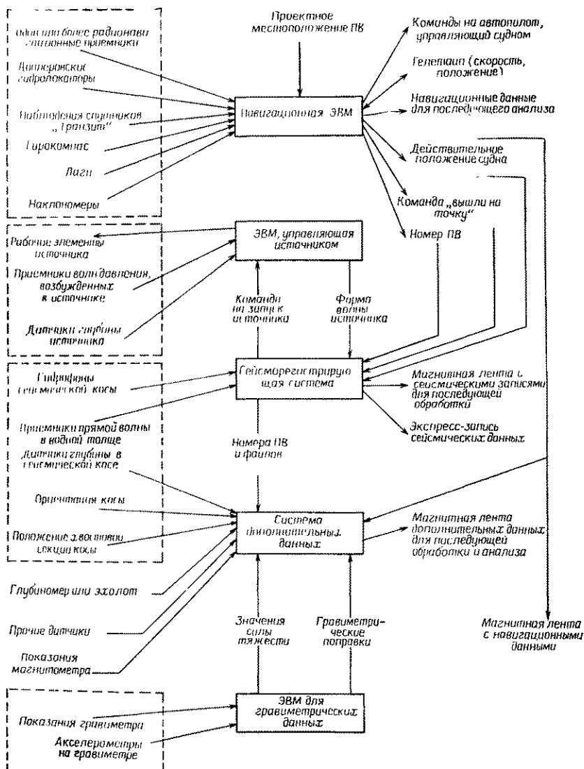
Рис. 5.54. Блок-схема организации потока данных при морских исследованиях. Отдельными кораблями не обязательно используются все приборы, приведенные на схеме, соединение устройств также может несколько отличаться [185].
