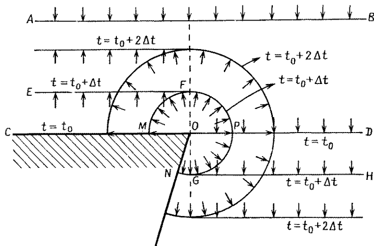
Рис. 2.24. Фронты волн, испытавших дифракцию от пласта, нарушенного сбросом.
