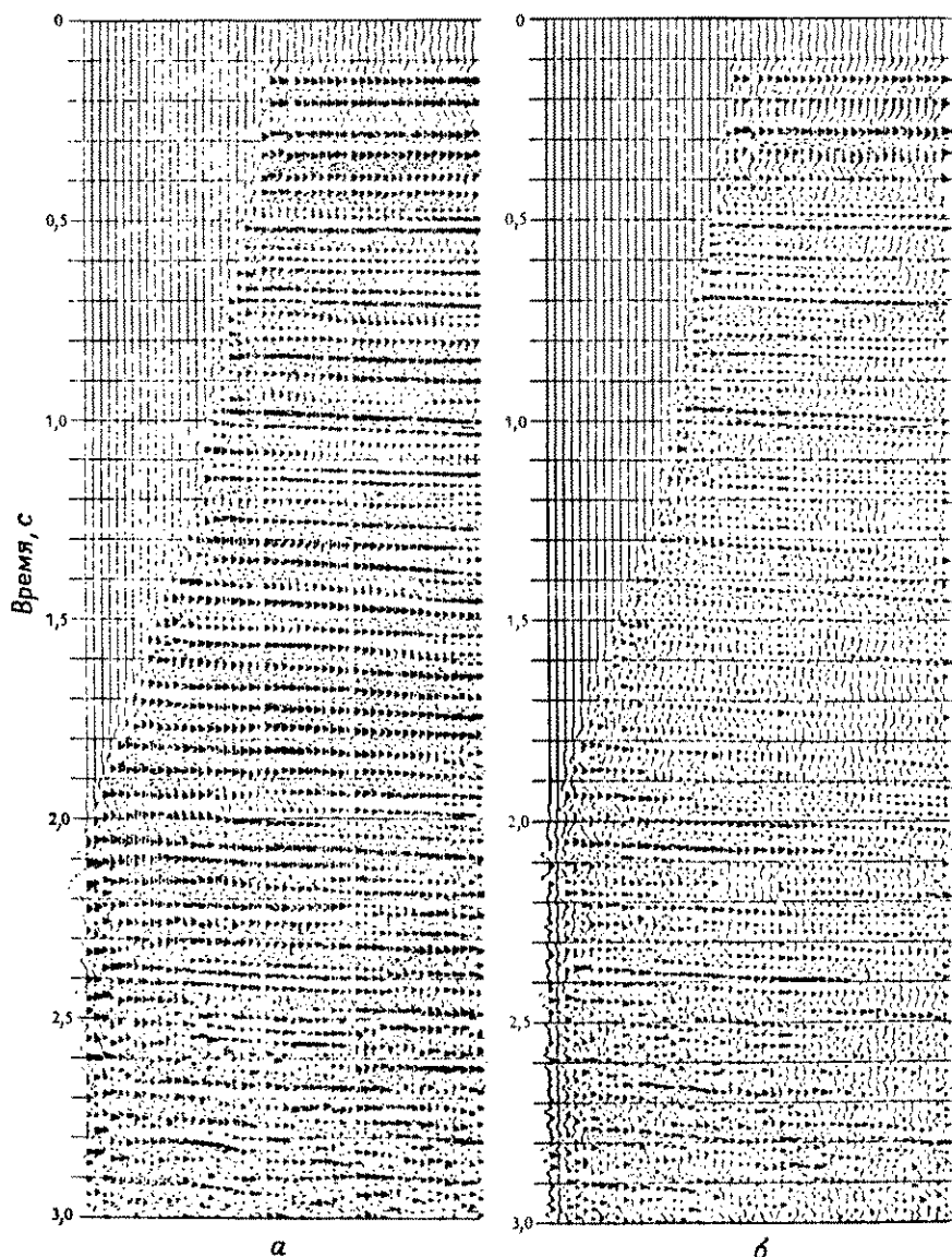
Рис. 4.12. Сейсмическая запись многократных отражений в неглубоком слое воды («поющая» запись). [С разрешения «Петти-Рей джеофизикал»]. а — полевая запись; б — то же после деконволюции, устраняющей этот эффект (§ 8.1.2г).
