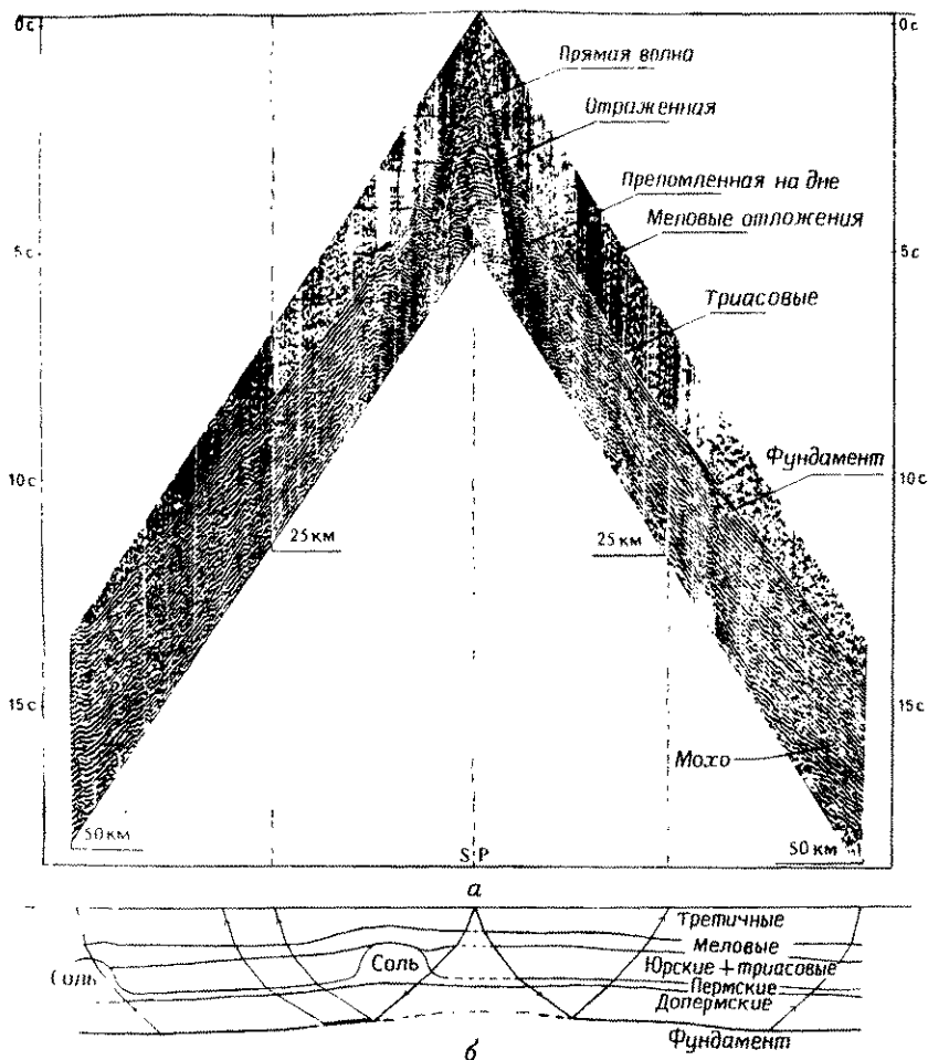
Рис. 6.10. Разрез МПВ. [С разрешения «Пракла-Сейсмос»] а — временной разрез; б — геологический разрез.
