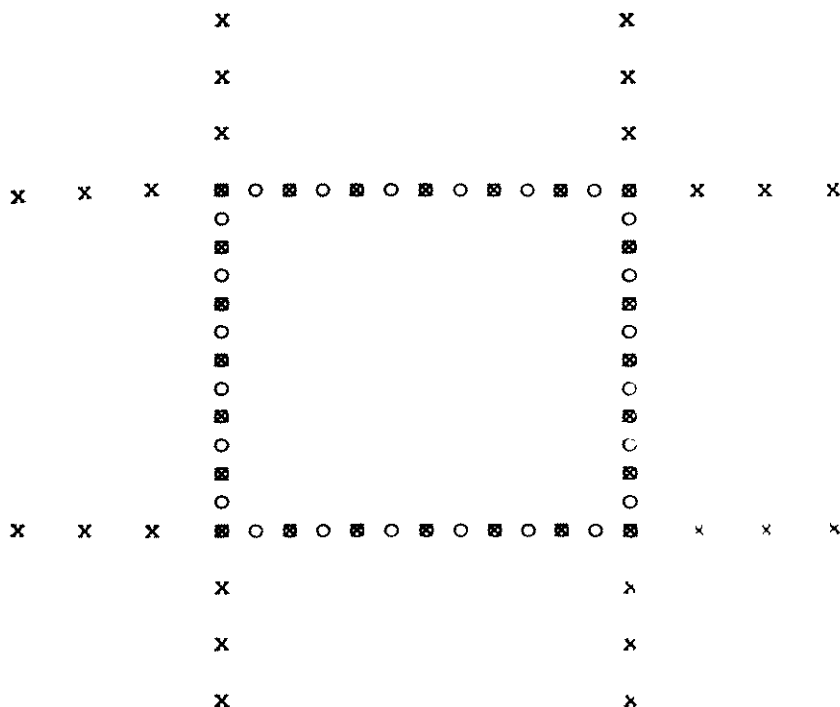
Рис. 5.69. Схема трехмерных наблюдений. Положения пунктов взрыва показаны крестиками, центров групп сейсморегистраторов — кружками.
