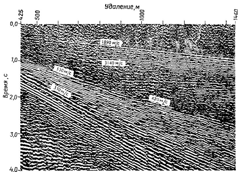
Рис. 5.14. Анализ волн-помех [179]. Сейсмоприемники разнесены на 1,5 м, удаление первого приемника 425 м. Проведена следующая идентификация волн по скоростям: 1890 м/с — волна, преломленная в подошве ЗМС; 530 и 620 м/с — моды поверхностных волн; 330 м/с — звуковая воздушная волна; 3140 м/с — преломленная волна.
