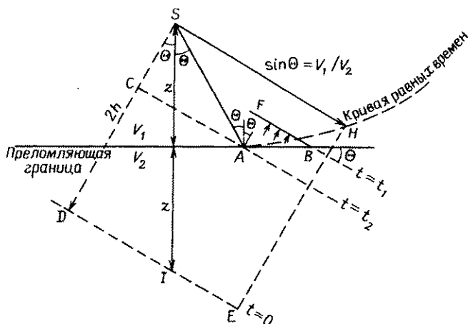
Рис. 6.22. К выводу свойств кривой совпадения (т. е. равных) времен.
