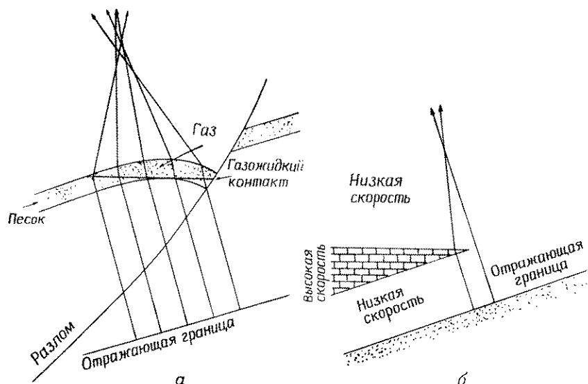
Рис. 4.20. Фокусировка лучей за счет изменений скорости. а — низкая скорость в газовой залежи создает эффект погребенного фокуса для более глубоких отражений; б — выклинивание высокоскоростного слоя создает эффект погребенного фокуса.
