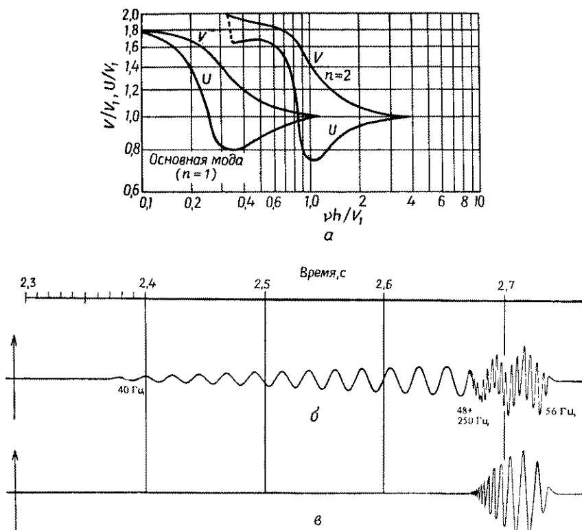
Рис. 2.30. Распространение нормальных мод. а — зависимости фазовой и групповой скоростей от нормированной частоты в случае жидкого слоя, залегающего на упругом субстрате, когда a_2/a_1 = 2\sqrt{3} , \sigma_1 = 0,5 , \sigma_2 = 0,25 , \rho_2/\rho_1 = 2,5 [55]; б — волновой пакет для первой моды колебаний, возбужденных источником на расстоянии 4 км; в — высокочастотная часть пакета б, называемая водной волной ; ее первое вступление используется в работах МПВ для определения дистанции (см. задачу 3.14) [40].
