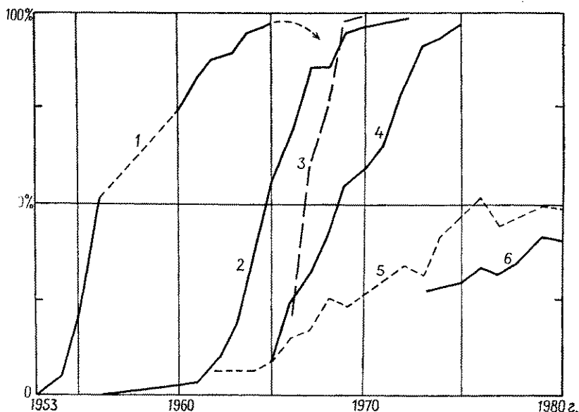
Рис. 1.20. Доля различных видов сейсмических работ в общем объеме сейсморазведки в США. (Данные из годовых отчетов SEG о геофизических работах.) 1 — аналоговая магнитная запись, 2 — метод ОГТ, 3 — морская сейсморазведка без динамита, 4 — цифровая регистрация, 5 — поверхностные источники на суше, 6 — Вибросейс.
