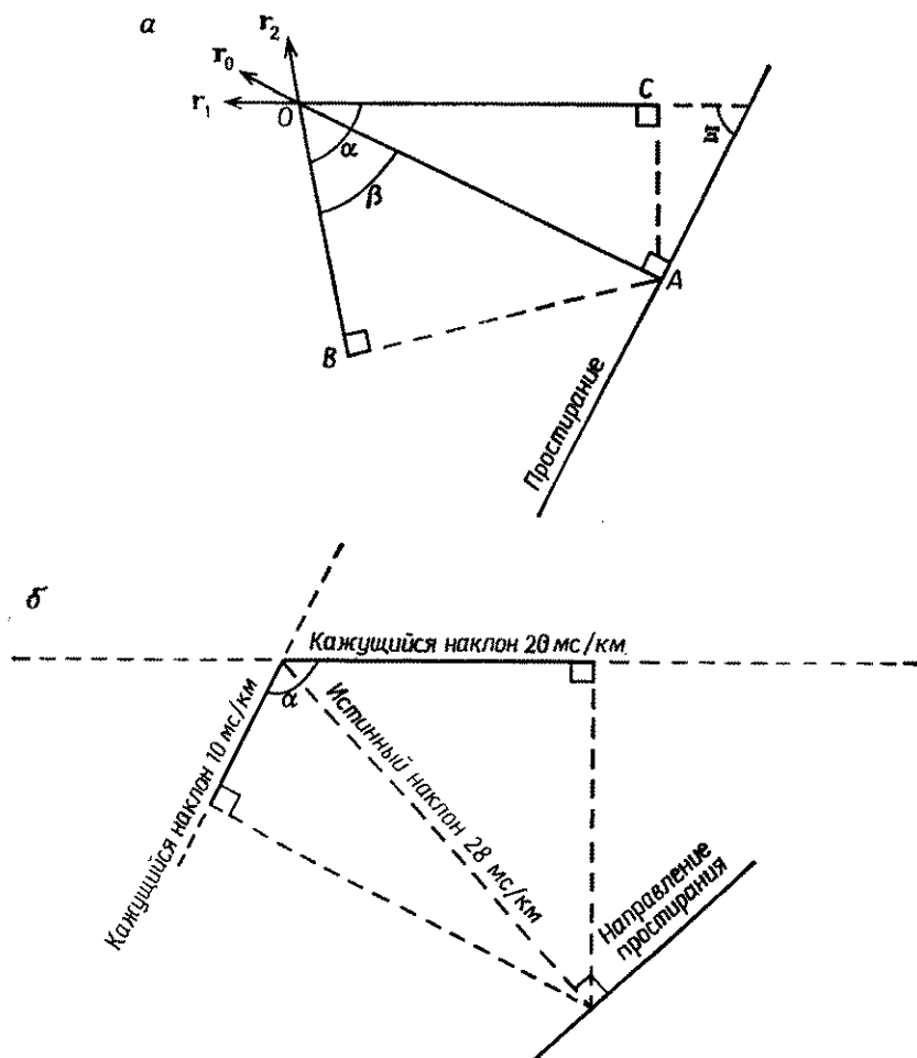
Рис. 3.8. Определение углов падения и простираия, когда линия наблюдений не перпендикулярна простираию пласта. а — связь между точкой наблюдения O и точкой отражения A (точка A всегда смещена по восстанию относительно точки O ); б — пример графического решения.
